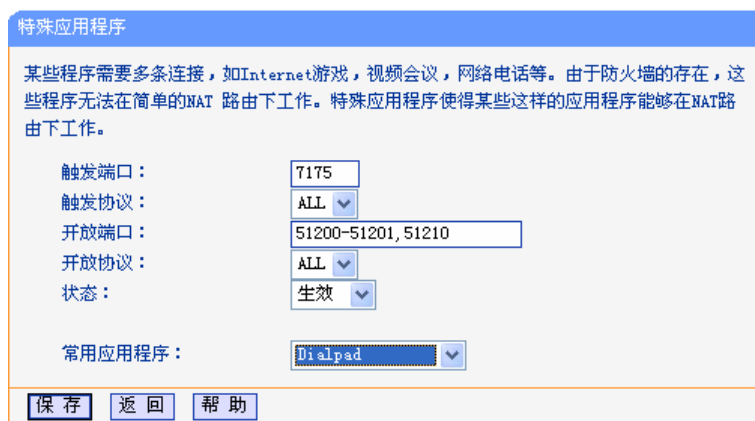
图 5-29 设置特殊应用程序条目
