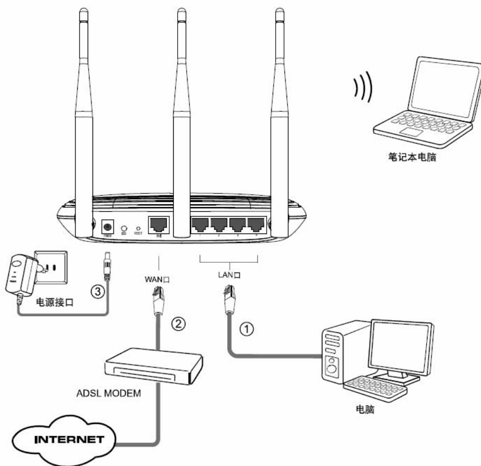
图 4-1 TL-WR941N 硬件安装示意图
