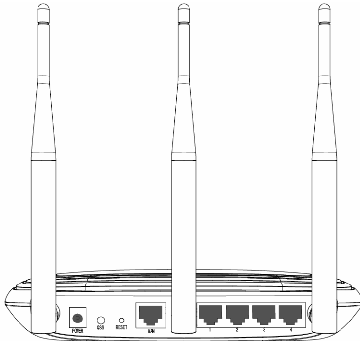
图 3-2 TL-WR941N 后面板示意图
